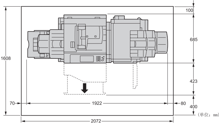
带有C1 型骑马马装订器（选装）和侧接收盘（选装）
