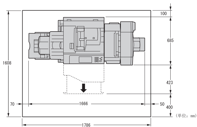
带有完成装订部 B1 用小册子装订组件 (选装) 和侧接收盘 (选装)
