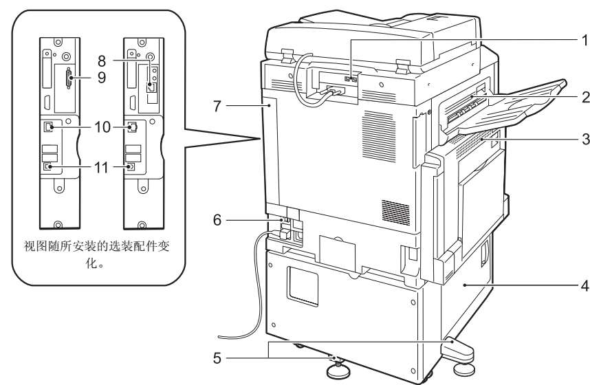
■机器的左侧和背面视图
