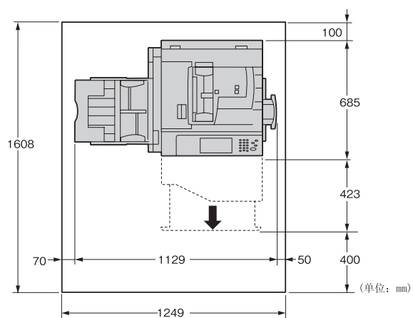
带有完成装订部 A1 (选装)
