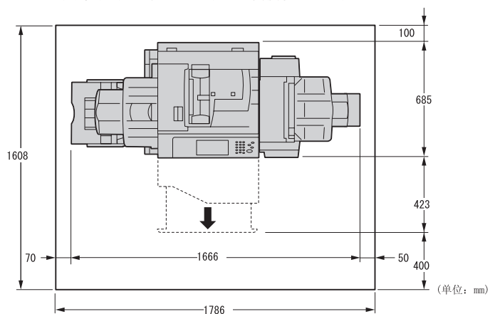
带有完成装订部 B1 (选装) 和侧接收盘 (选装)
