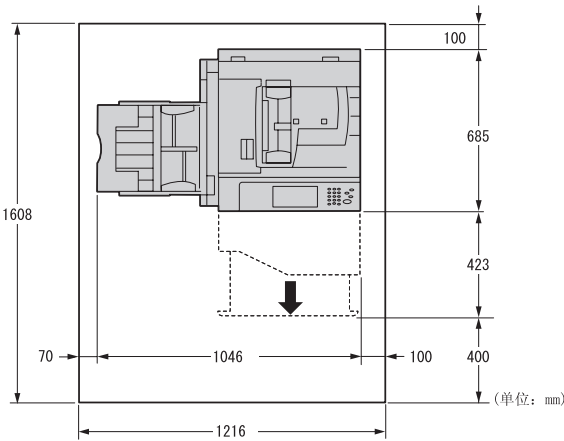
带有自动双面输稿器（选装）
