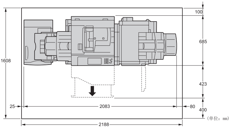
带有完成装订部C1（选装）、大容量纸盘B1（选装）和侧接收盘（选装）
