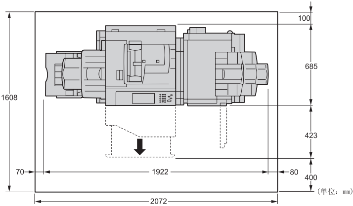
带有完成装订部 C1（选装）和侧接收盘（选装）
